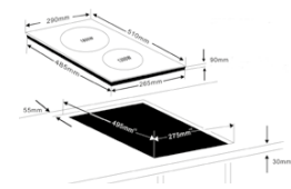
Posibilidad de encastrar Encastrable option
