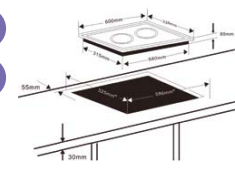
Posibilidad de encastrar Encastrable option
