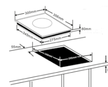
Posibilidad de encastrar Encastrable option
