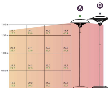
Área de calentamiento · Heating area
