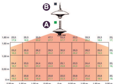
Área de calentamiento · Heating area
