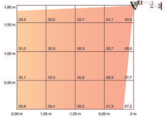
Área de calentamiento · Heating area
