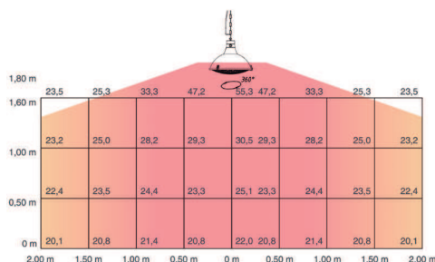
Área de calentamiento · Heating area
